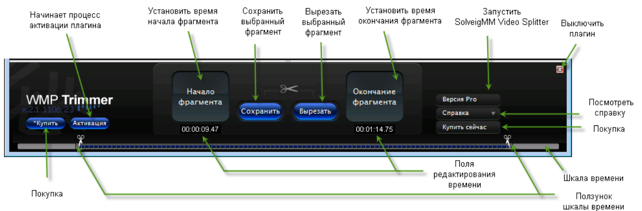
Рис. 4. Элементы управления плагина SolveigMM WMP Trimmer (подробное изображение)
